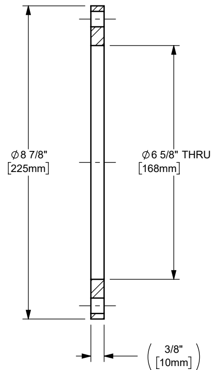
SECTION A-A
